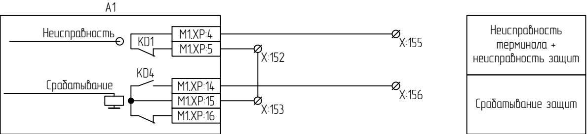
Цепи PAC
