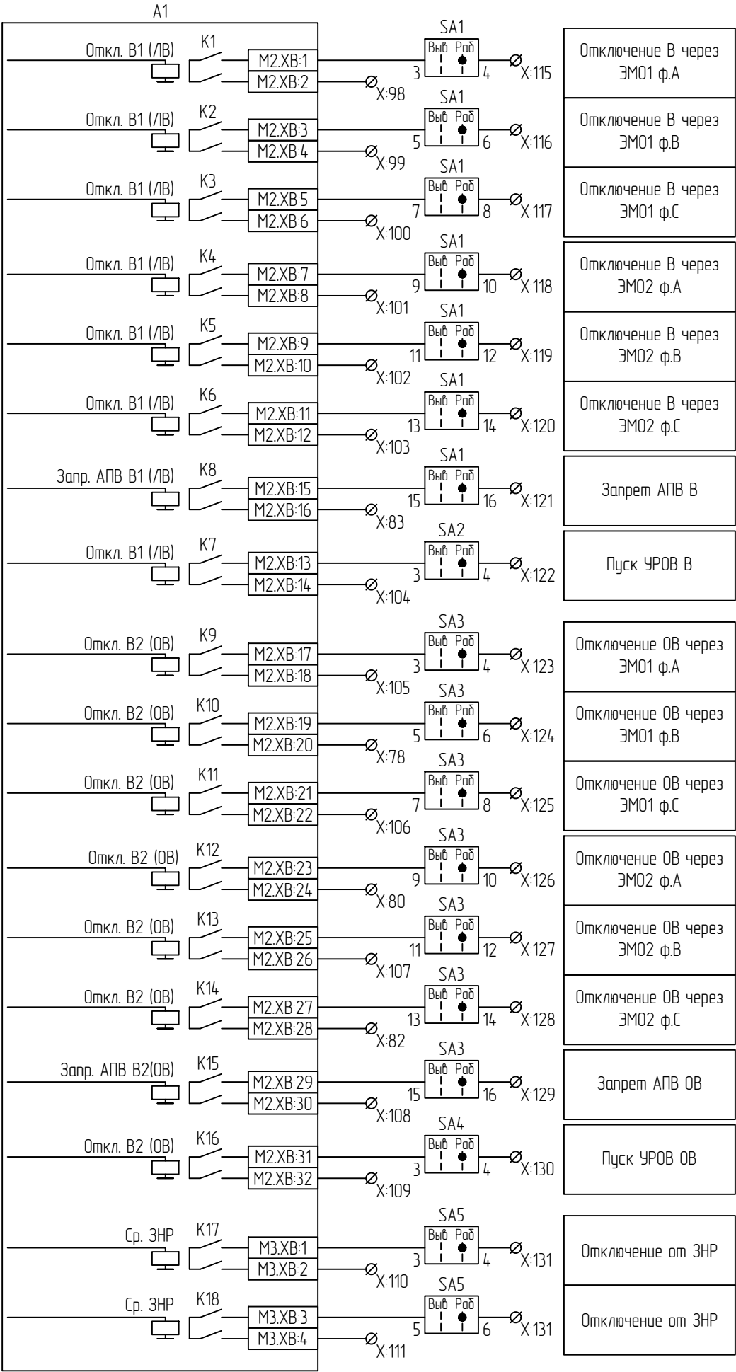
Выходные цепи
